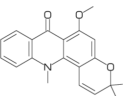
[55] Acronycine
