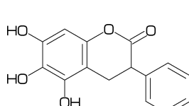
[63] Baicalein
