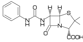
[43] Gibberellin A3
