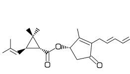
[67] Pyrethrin I
