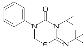
[31] Buprofezin
