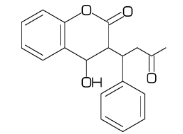
[66] Rotenone
