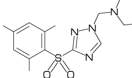
[28] Pendimethalin
