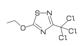
[11] Etridiazole
