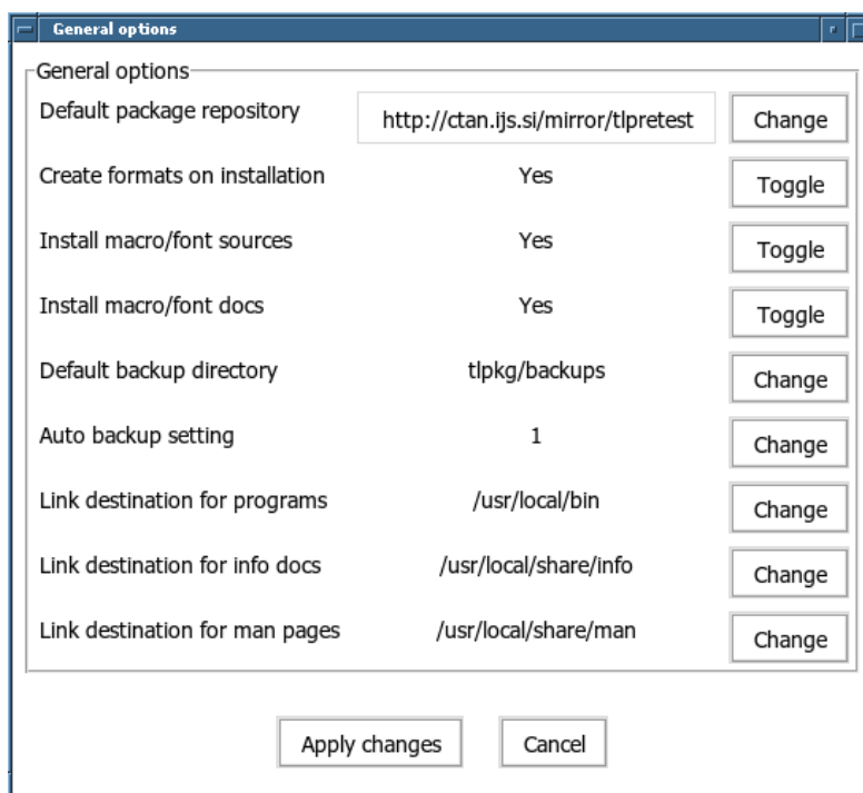
Abbildung 6.2: tlmgr im GUI-Modus: Allgemeine Optionen
