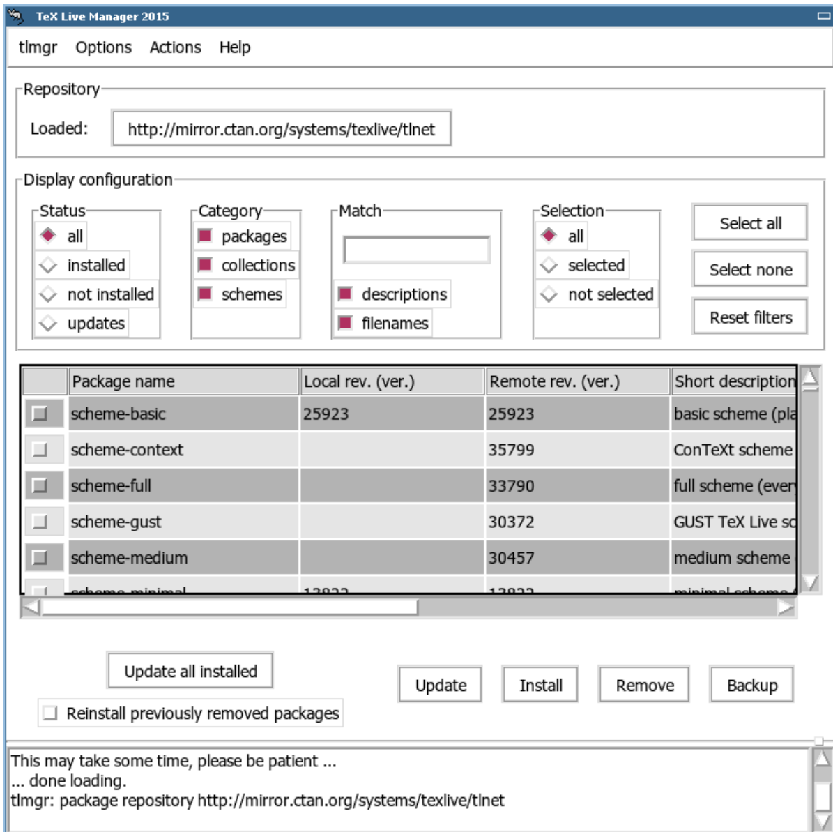
Abbildung 6.1: tlmgr im GUI-Modus. Hauptfenster nach dem Klicken auf »Load«.
