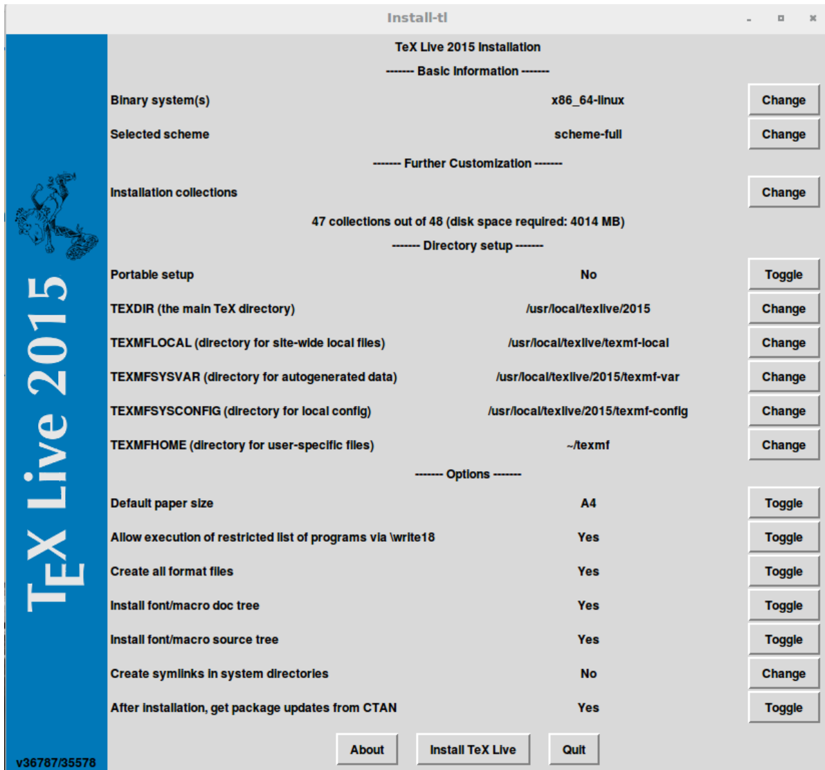
Рис. 3: Главное меню программы установки в экспертном графическом режиме (GNU/Linux)
