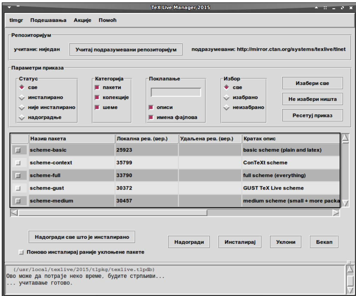
Слика 9: tlmgr у графичком (GUI) режиму рада: главни прозор, стање пре учитавања репозиторијума помоћу дугмета „Учитај“ („Load“).
